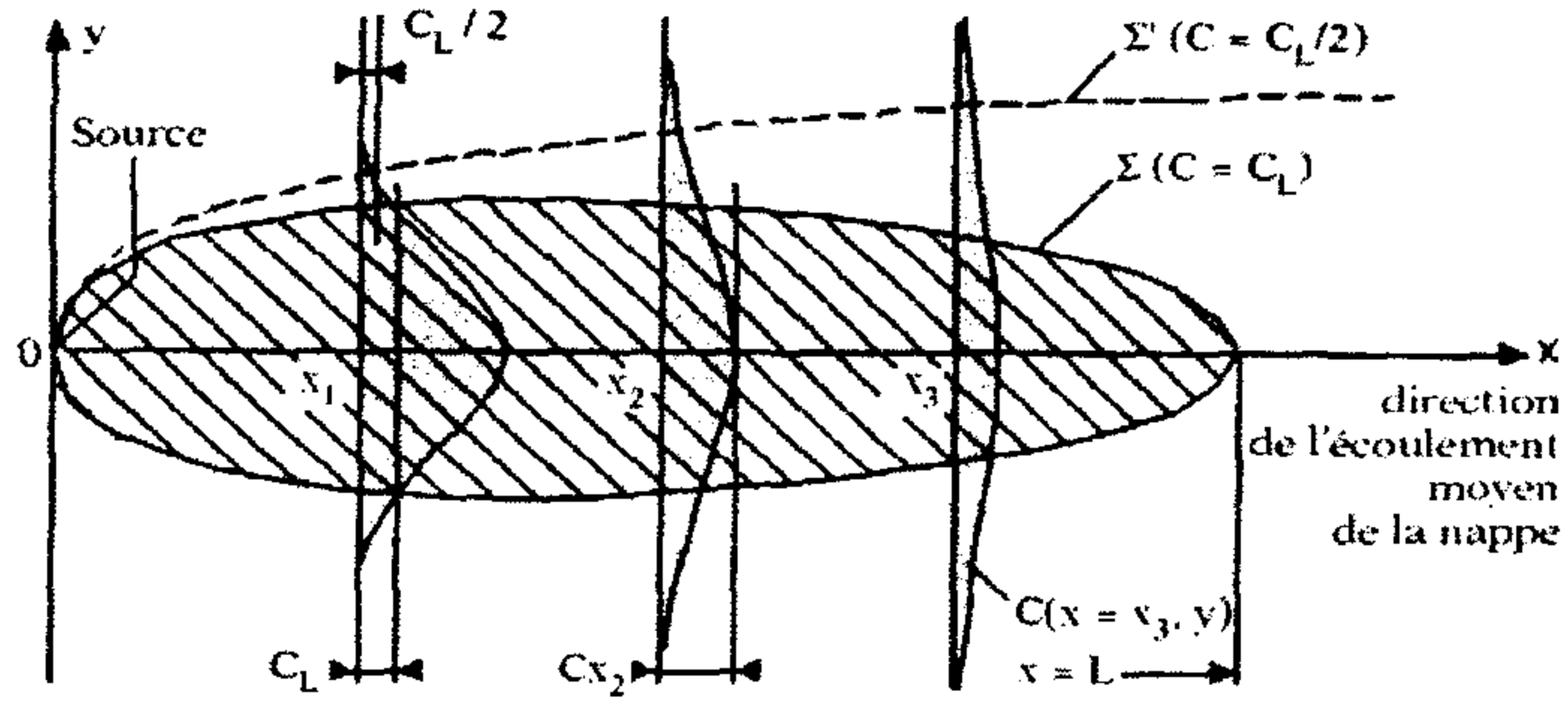
Délimitation du domaine contaminé : \Sigma(C = C_L) (ici, section longitudinale médiane du domaine tridimensionnel)
